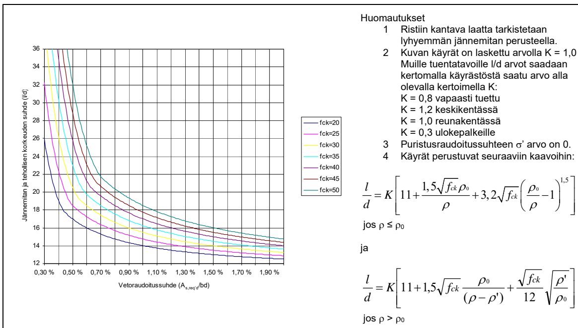
Kuva 4. Jännemitan ja tehollisen korkeuden rajasuhde
