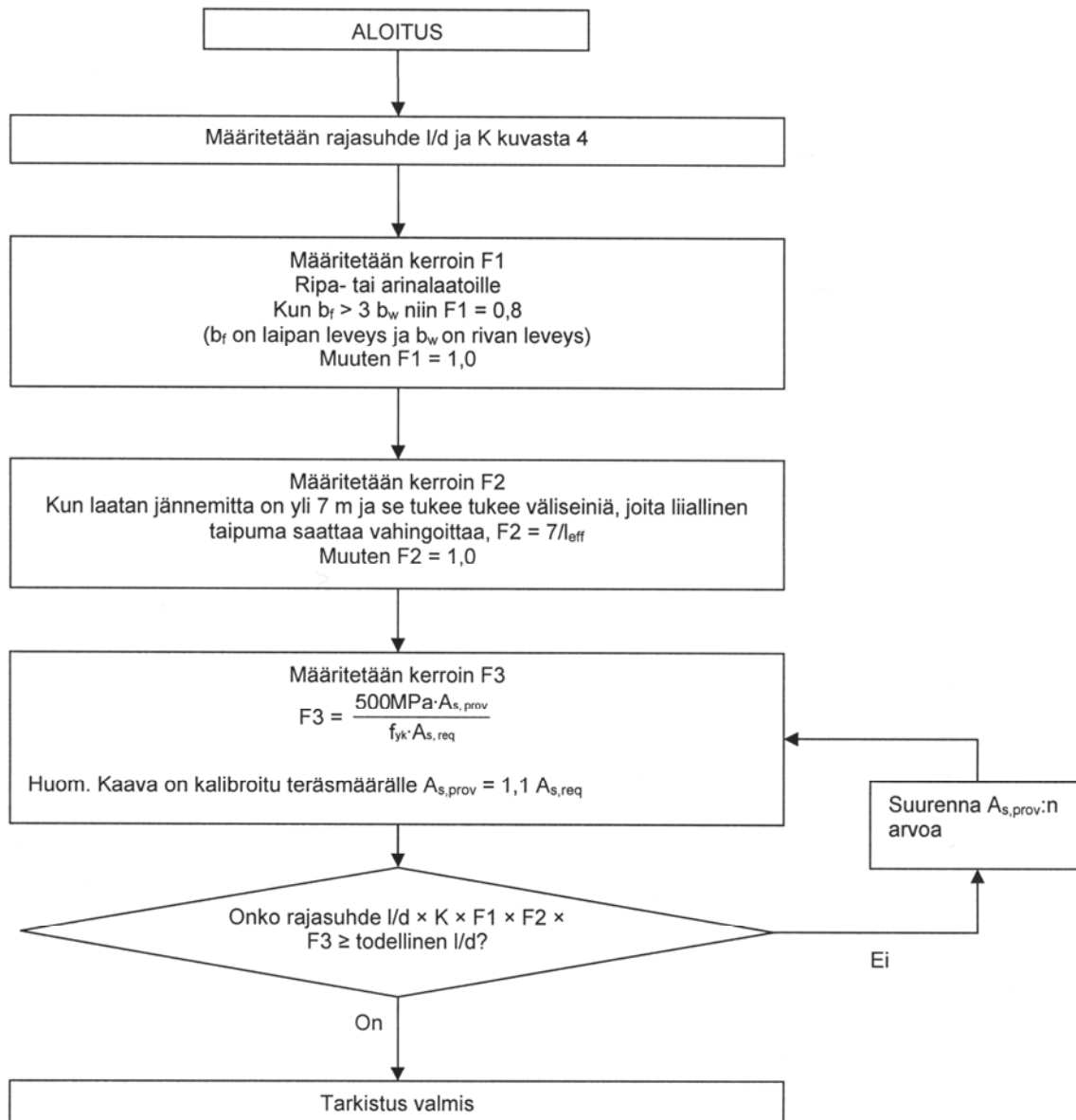
Kuva 3 Taipuman arviointimenettely
