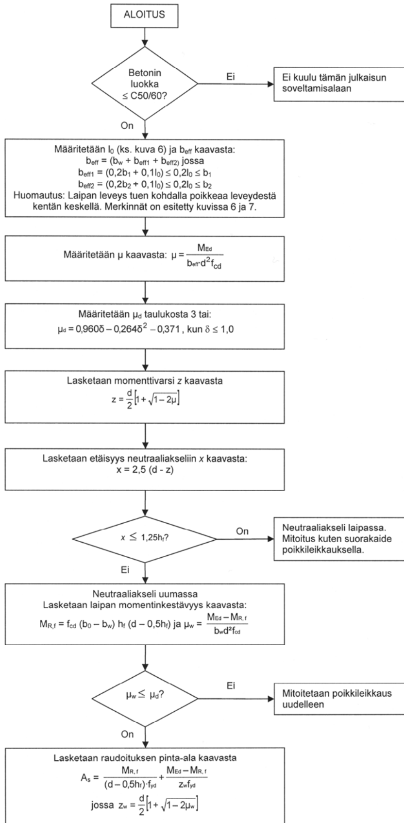
Kuva 5 Ripalaatan taivutuskestävyyden määrittäminen
