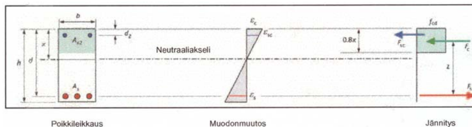
Kuva 2. Yksinkertaistettu suorakaiteen muotoinen jännitysjakuma eurokoodin EN 1992-1-1 mukaisesti, kun betonin lujuusluokka on korkeintaan C50/60.
